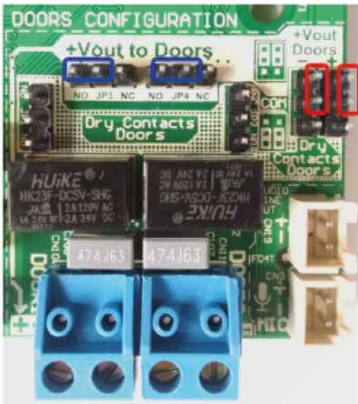
Salida con tensión Relé 1: NO Relé 2: NO
