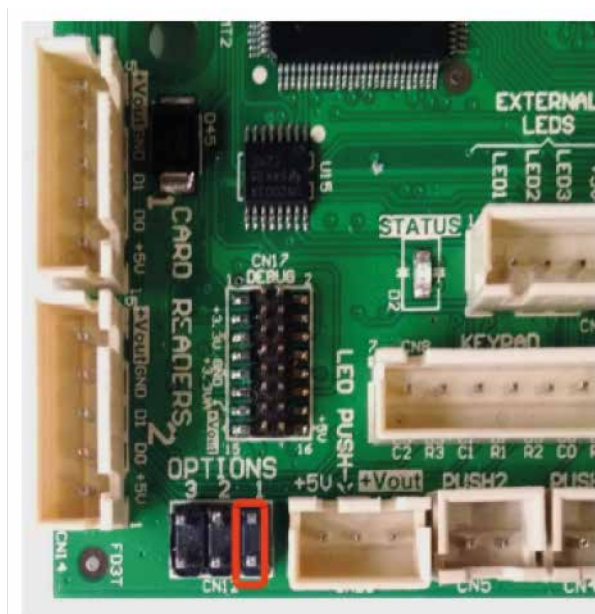
Figura 13 – Pines de configuración para forzar al equipo a su valor de IP de fábrica.
