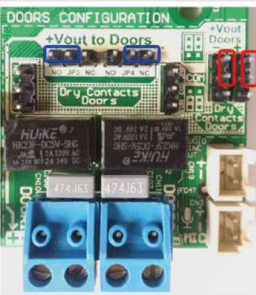
Salida con tensión Relé 1: NO Relé 2: NC
