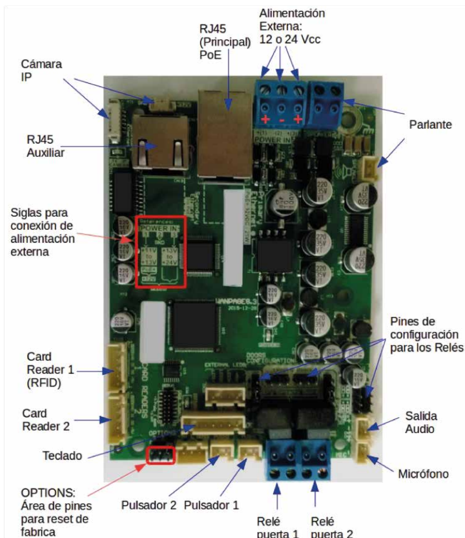
Figura 10 – Placa electrónica de IP Access con videocámara
