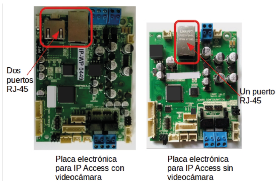
Figura 9 – Modelos de placa electrónica de IP Access
