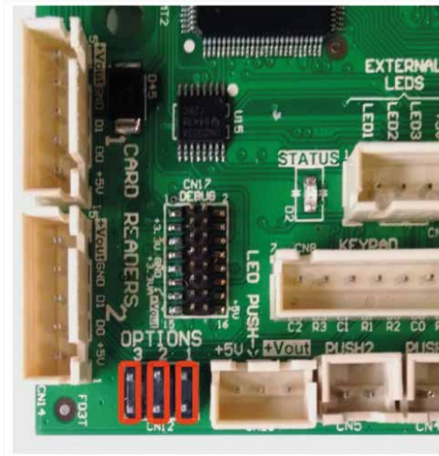
Figura 14 – Pines de configuración para forzar al equipo a los valores de fábrica.
