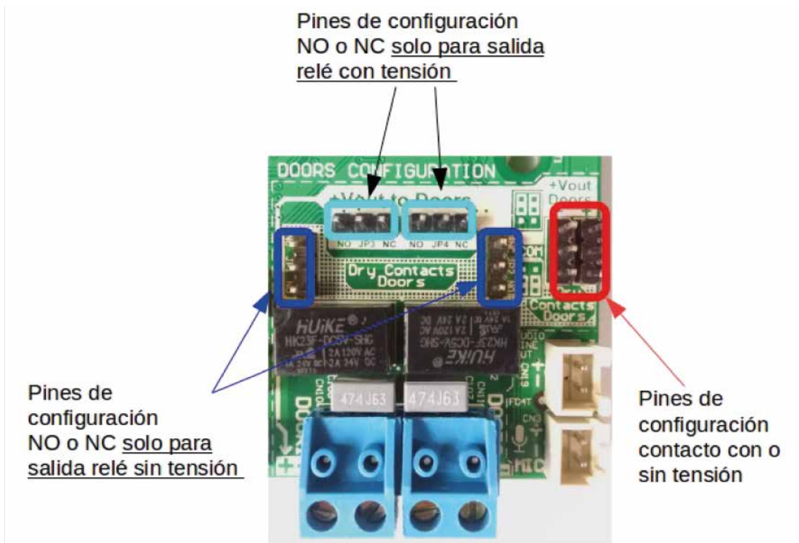
Figura 12 – Área de pines de configuración de relé
